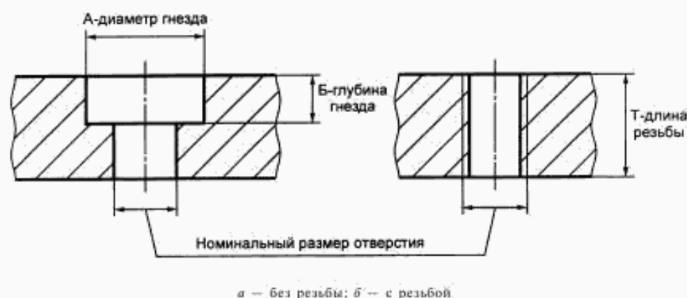
Рисунок 1 — Вспомогательные отверстия для крепления дополнительных деталей и устройств на корпусах и крышках задвижек
